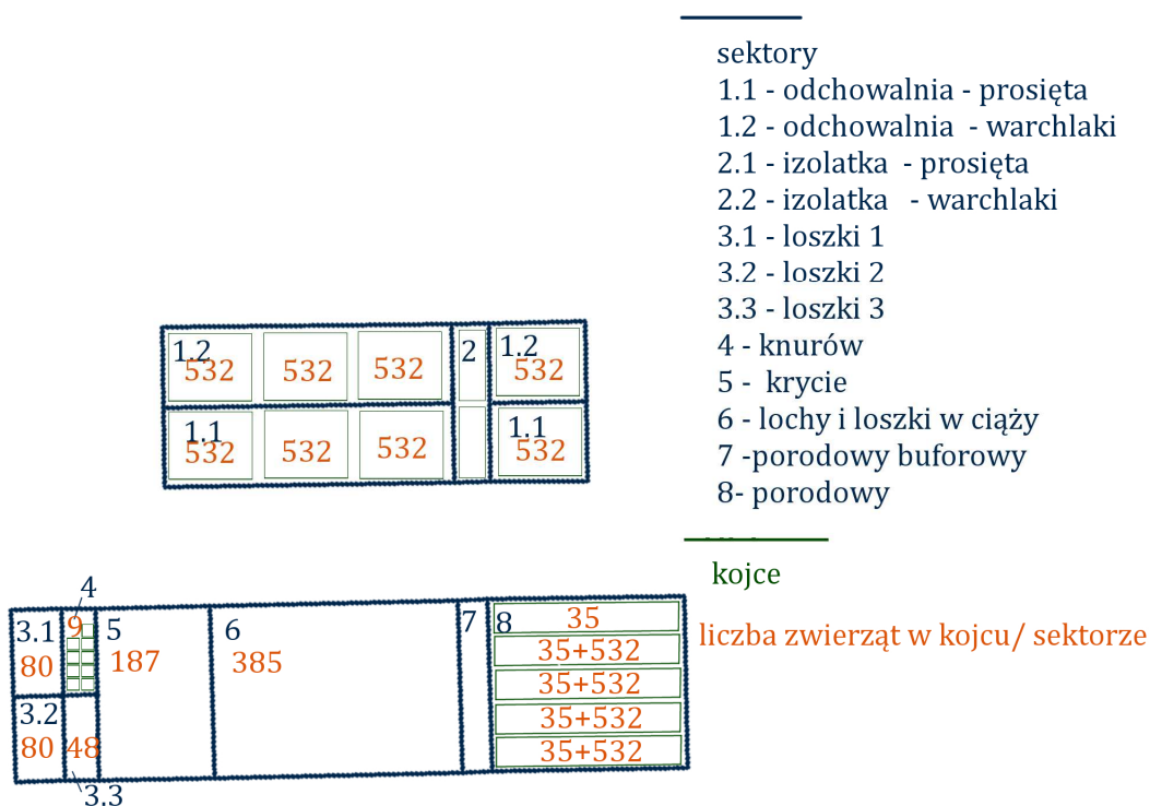
Rysunek 1 Schemat stada technologicznego
